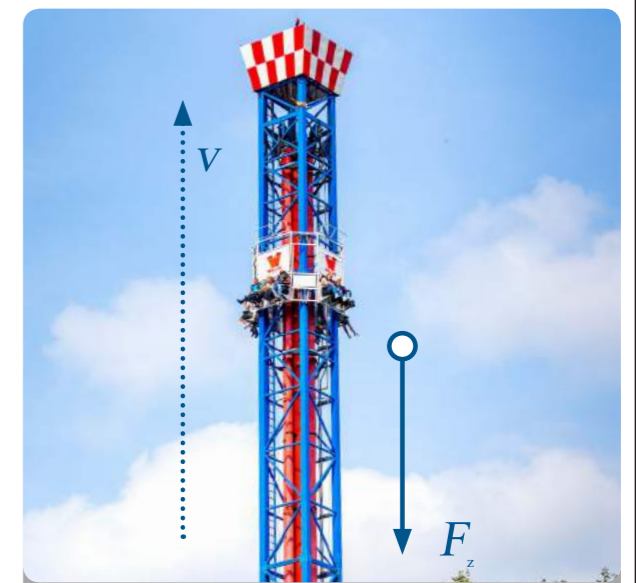
FIG. 4.20 Vertraagde beweging omhoog.
