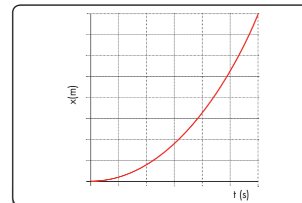
FIG. 2.8 Het (x,t) -diagram van een wandelaar.
