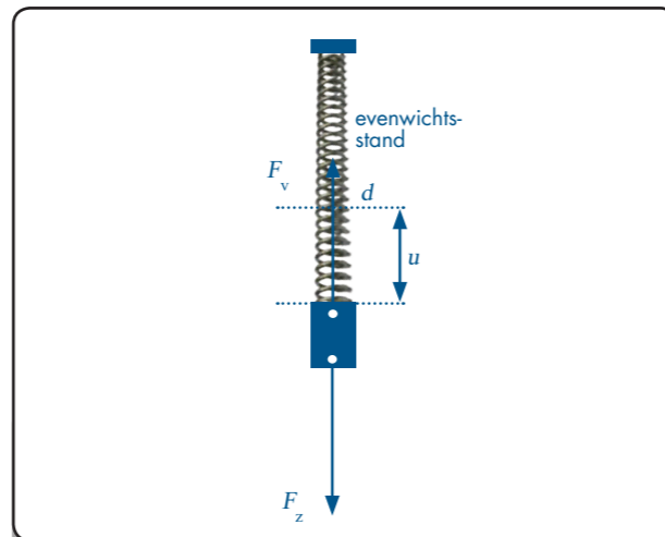
FIG. 4.16 Krachten op een veer.
