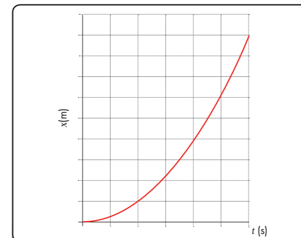
FIG. 2.18 (x,t) -diagram van een versnelde beweging.
