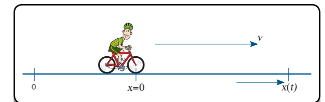
FIG. 2.14 Een fietser beweegt langs een lijn.
