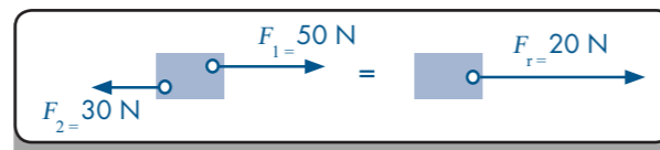
FIG. 4.8 Krachten optellen die in tegengestelde richting staan.
