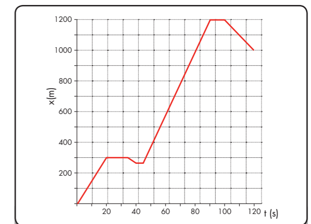
FIG. 2.10 (x,t) -diagram bij opgave 10.
