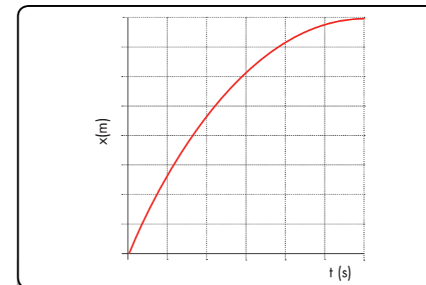
FIG. 2.9 Het (x,t) -diagram van een vertraagde beweging.
