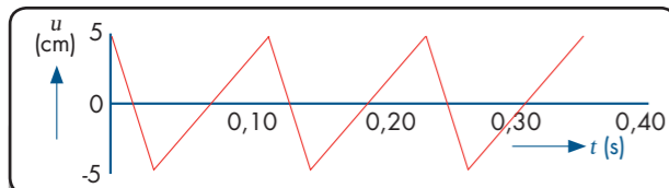
FIG. 3.12 Een zaagtandvorming ( u, t )-diagram.
