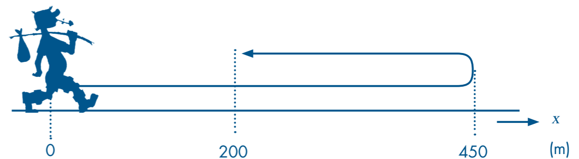
FIG. 2.2 Verplaatsing en afgelegde weg.
