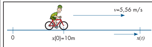
FIG. 2.15 Een fietser rijdt met een constante snelheid van 20 km/uur.
