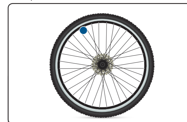
FIG. 3.6 Een draaiend fietswiel.
