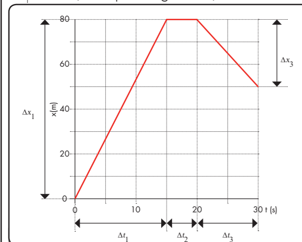
FIG. 2.7 Het (x,t) -diagram van een wandelaar.
