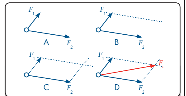
FIG. 4.9 Krachten optellen die in een willekeurige richting staan.
