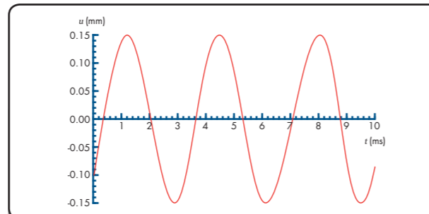
FIG. 3.13 Een ( u, t )-diagram (van een harmonische trilling).
