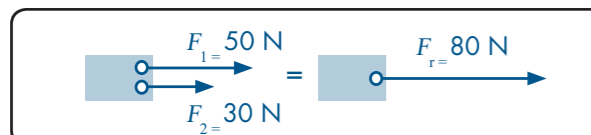
FIG. 4.7 Krachten optellen die in dezelfde richting staan.
