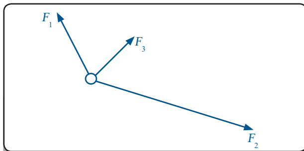
FIG. 4.12 Op een voorwerp werken drie krachten.
