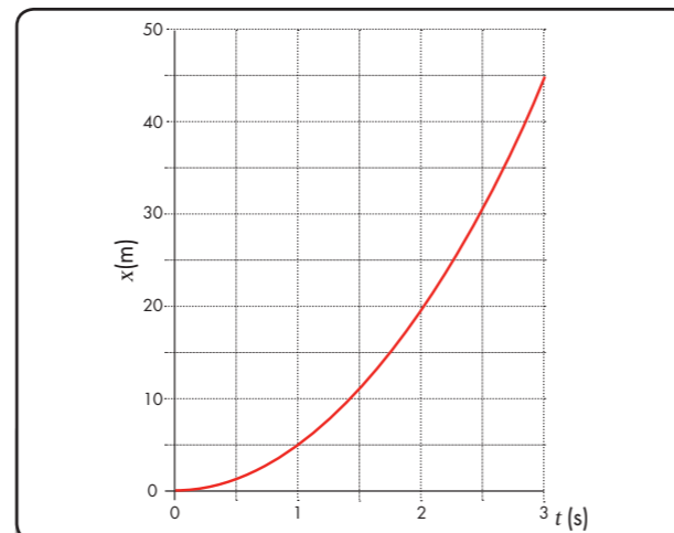
FIG. 2.12 (x,t) -diagram bij opgave 12.
