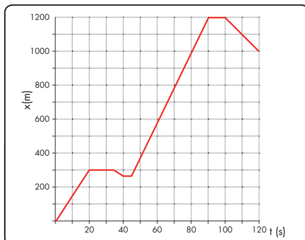
FIG. 2.11 (x,t) -diagram bij opgave 11.
