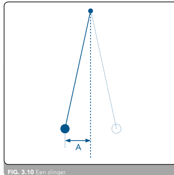
FIG. 3.10 Een slinger.
