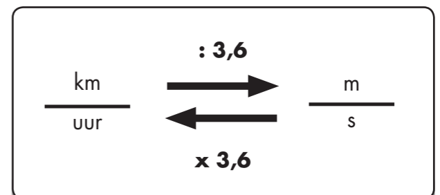
FIG. 2.5 Omrekenen van snelheid.
