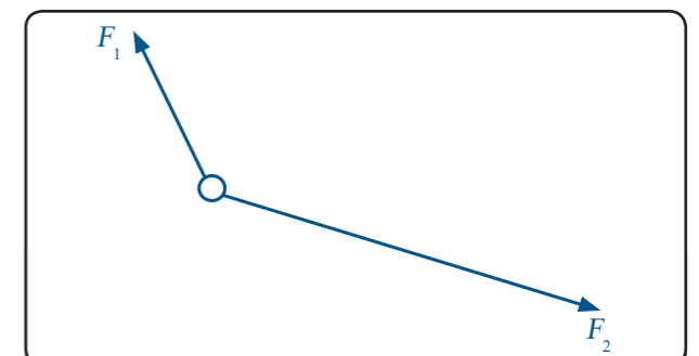
FIG. 4.10 Op een voorwerp werken twee krachten.
