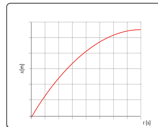
FIG. 2.19 (x,t) -diagram van een vertraagde beweging.
