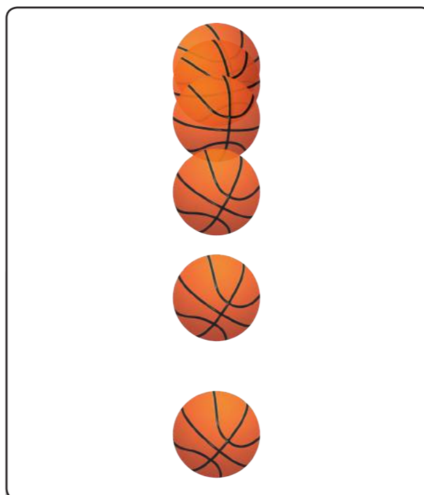
FIG. 3.1 Een vallende bal.
